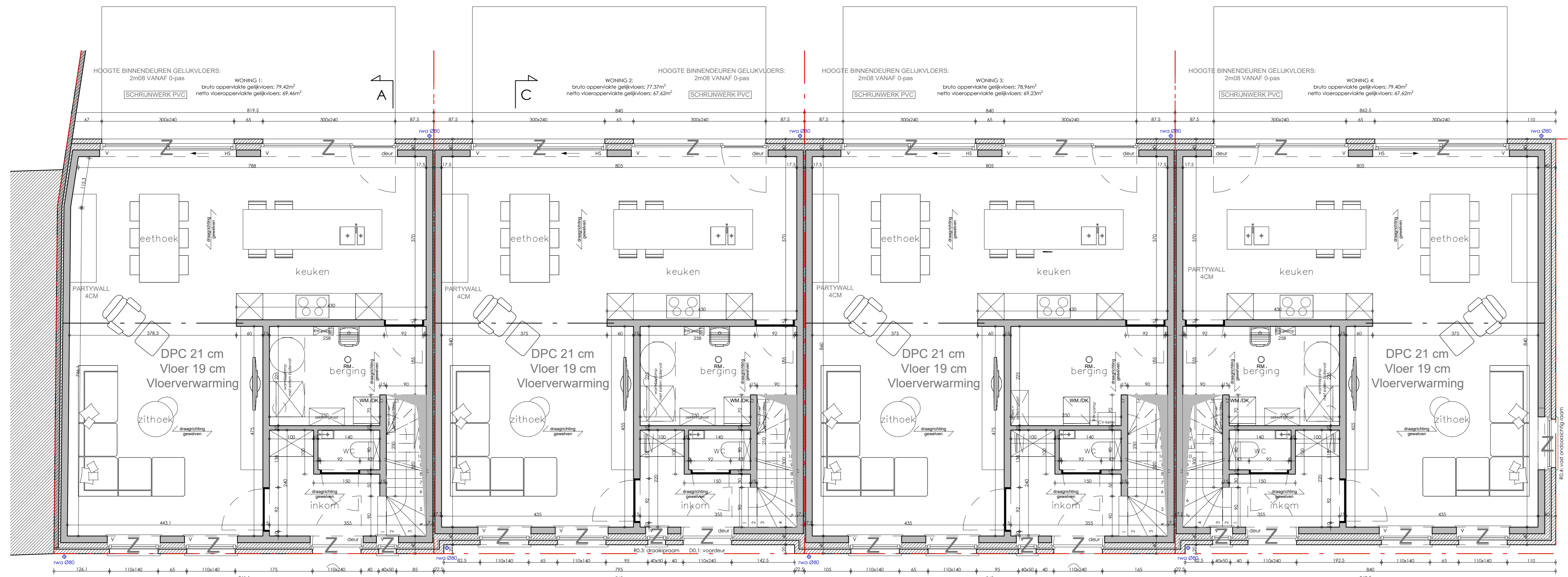
GELIJKVLOERS Schaal 1:50
